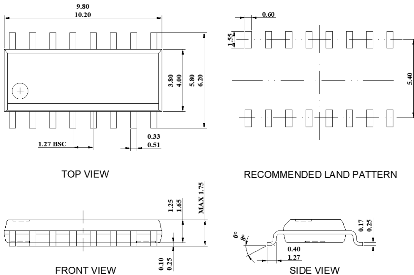
图 11- 2 SOIC16-NB(N)封装尺寸
