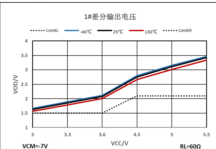
图 7-2 共模 -7V 时差分输出电压
