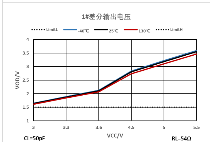
图 7-3 54Ω 负载下差分输出电压
