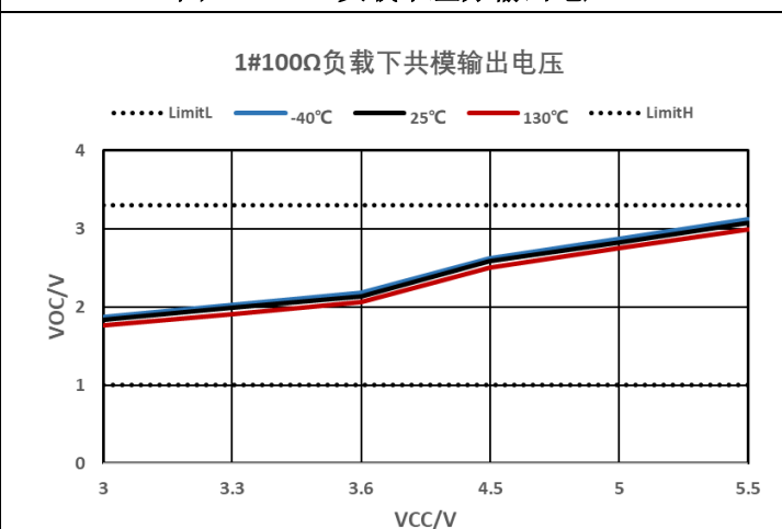
图 7-6 100Ω 负载下输出共模电压
