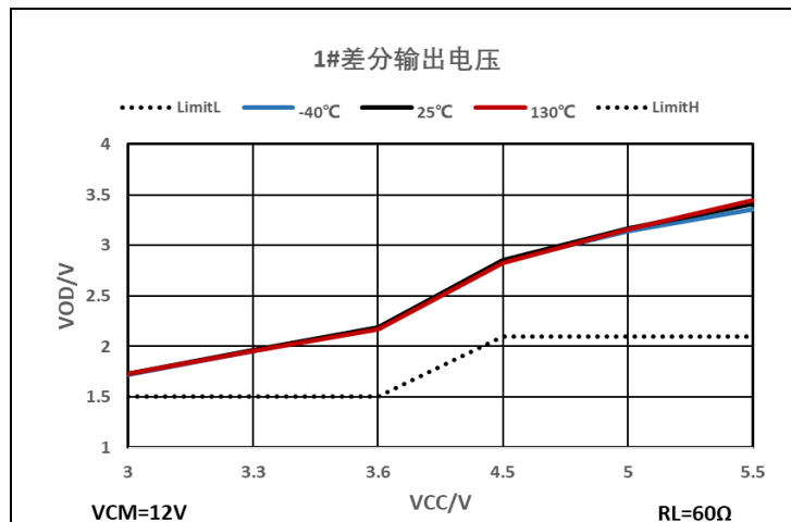
图 7-1 共模 12V 时差分输出电压
