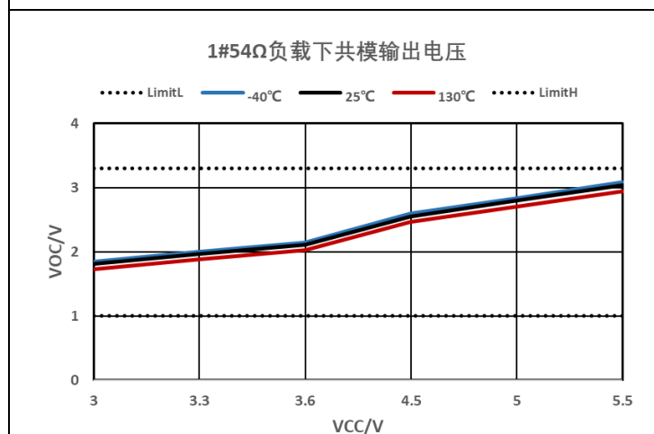
图 7-5 54Ω 负载下输出共模电压
