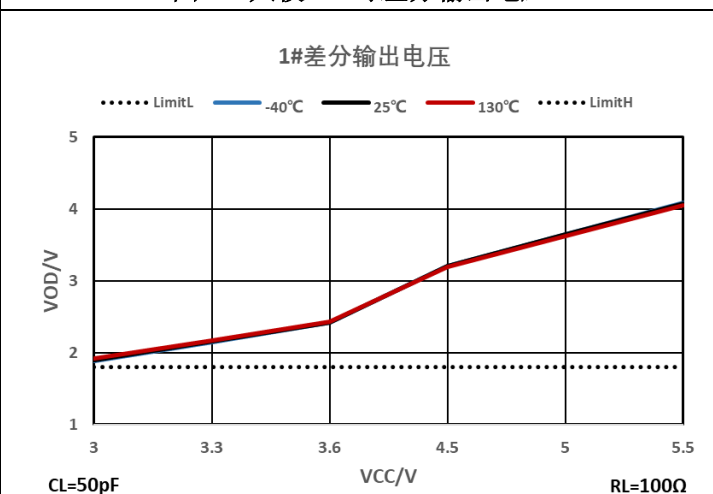
图 7-4 100Ω 负载下差分输出电压
